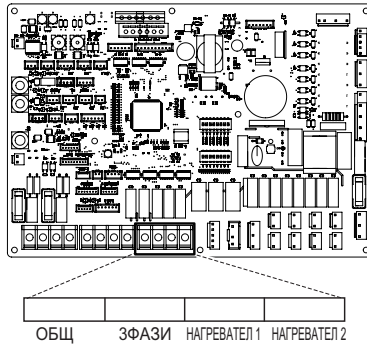
PCB на вътрешно тяло
