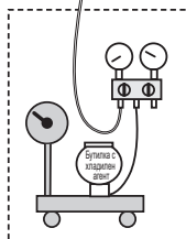
Двустраниен манометър Сервизен порт
